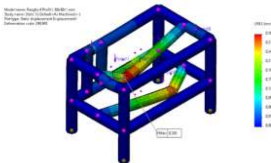
Hasil defleksi Maksimum Rangka Mesin Pengiris Tempe 40 x 40 x 1,5 mm
