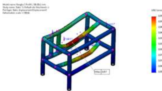
Hasil defleksi Maksimum Rangka Mesin Pengiris Tempe 40 x 40 x 1 mm
