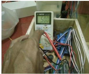
Gambar 3.6 Pengukuran ADC dengan NodeMCU (Sumber : Hasil Penelitian)
