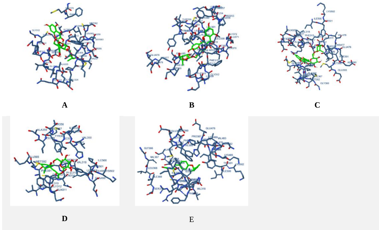
Gambar 2. Struktur ligan secara berturut - turut berikatan dengan PPAR \gamma yaitu (A) quercetin 3-O-neohesperidosid , (B) kaempfero 3-O-retinoside , (C) rutin , (D) roseoside , dan (E) Pioglitazon
