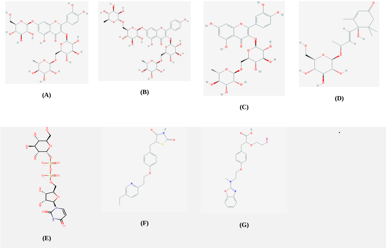
Gambar 1. Senyawa aktif daun Annona muricata Linn antara lain (A) quercetine 3-neohesperidoside , (B) kaempferol 3-O-rutinoside , (C) rutin , (D) roseoside , (E) Pioglitazon , (F) PPARγ , dan (G) Glikogen sintase
