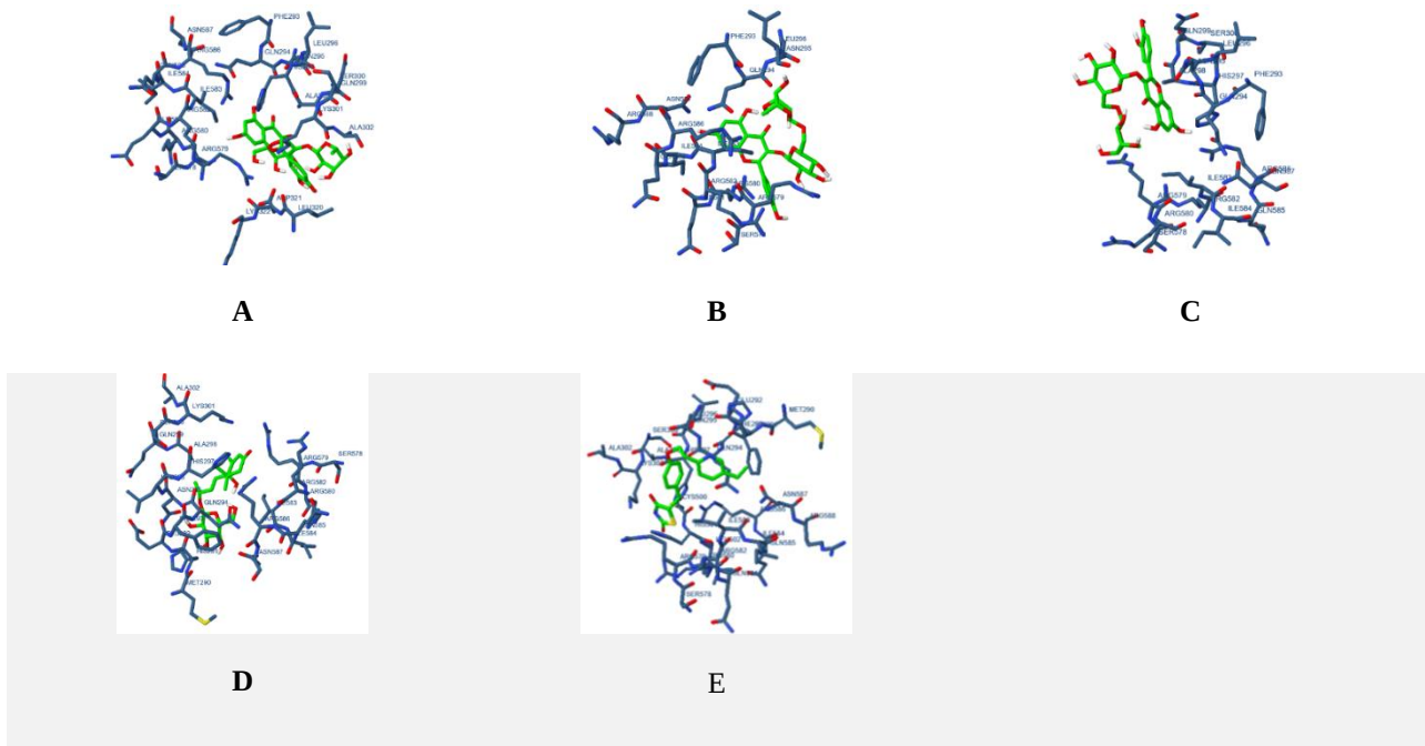
Gambar 3. Struktur ligan secara berturut - turut berikatan dengan glikogen sintase yaitu (A) quercetin 3-O-neohesperidoside , (B) kaempferol 3-O-rutinoside , (C) rutin , (D) roseoside , dan (E) Pioglitazon
