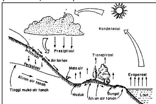
Gambar 1 Daur Hidrologi
