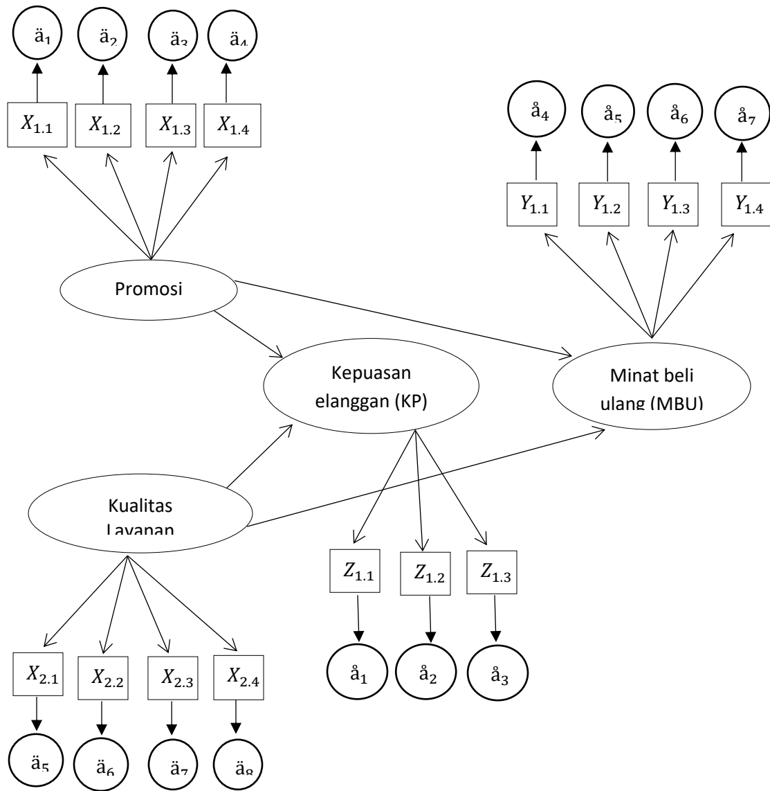
Gambar: Penyusunan Diagram Jalur untuk perancangan inner model dan outter model.
